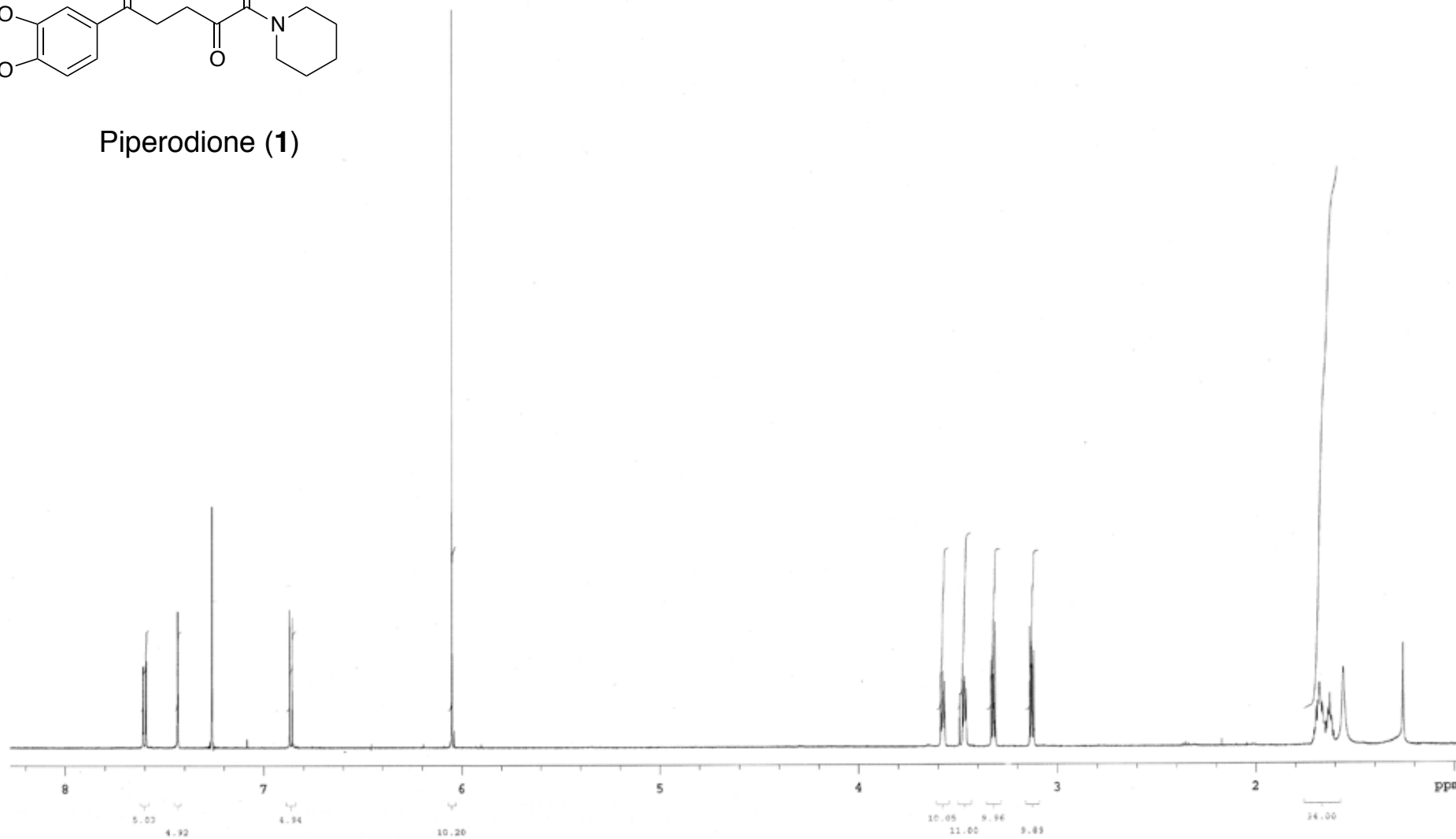
1 H NMR data of piperodione (1)
