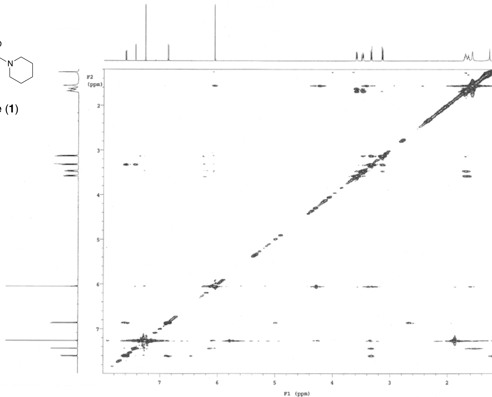
NOESY of piperodione ( 1 )
