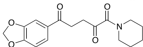
Piperodione ( 1 )
