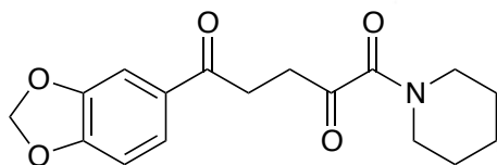
Piperodione (1)
