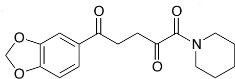
Piperodione (1)
