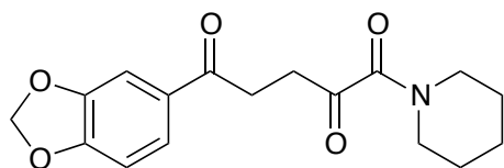
Piperone (1)
